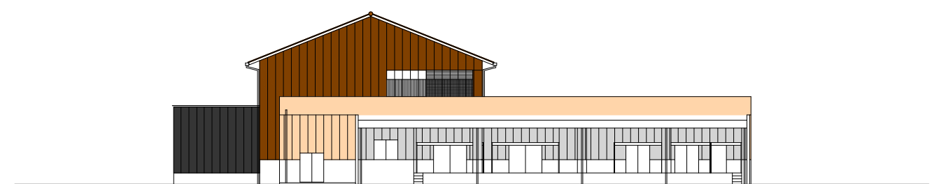
西面立面図
