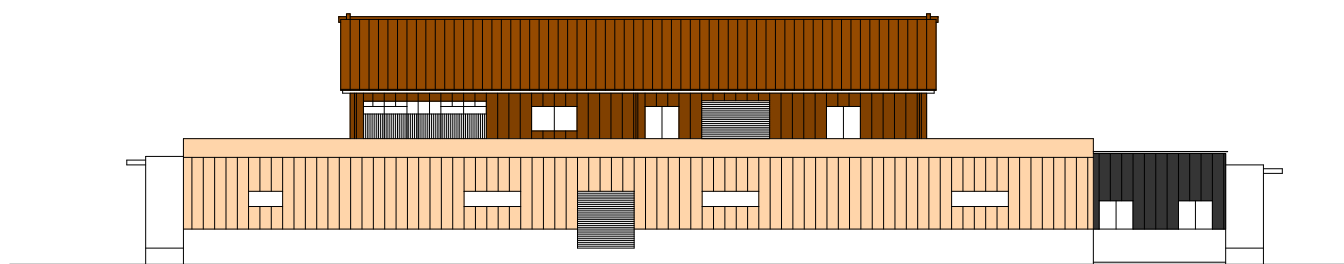
南面立面図
