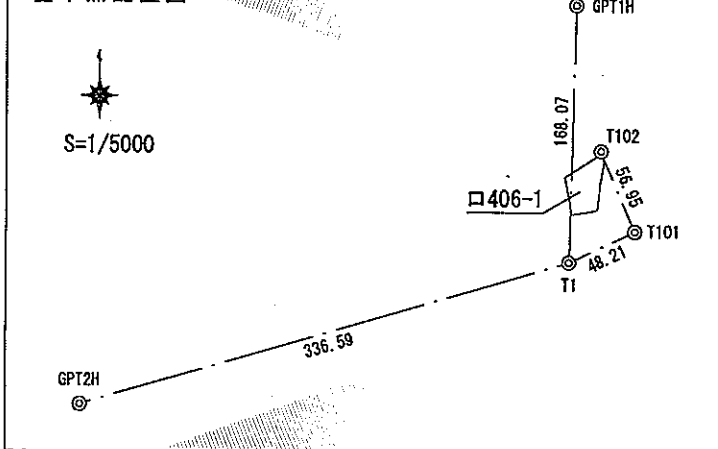
基準点配置図
